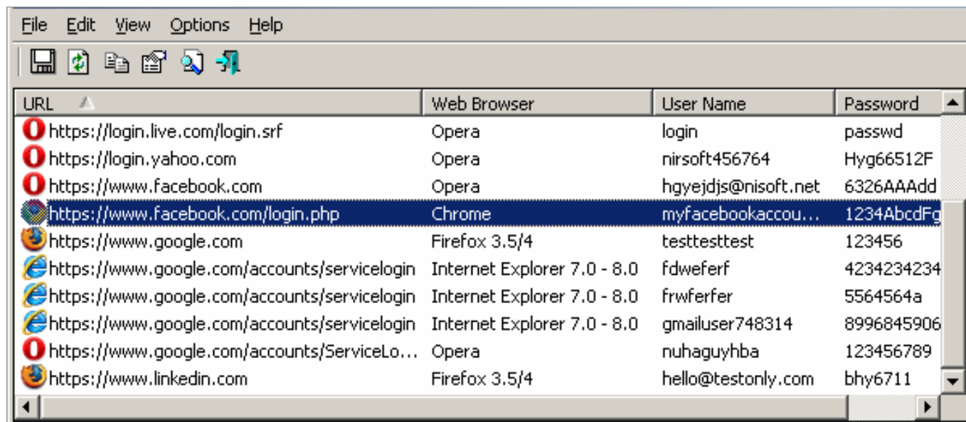
Рисунок 21: WebBrowserPassView
