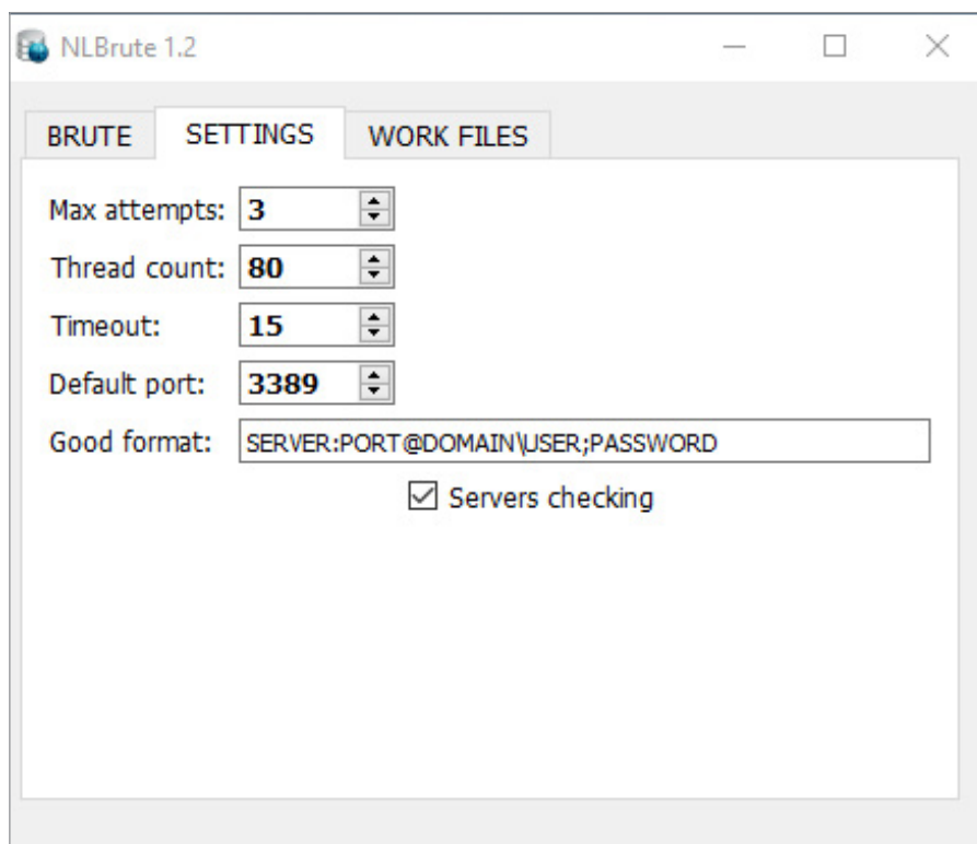
Рисунок 20: NLBrute 1.2
